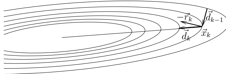
Abbildung 11: Ein Schritt der Methode der konjugierten Gradienten
