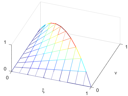
(d) \Phi_4(\xi, \nu) = 4\xi\nu
