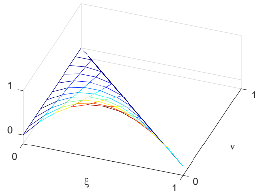
(f) \Phi_6(\xi, \nu) = 4\xi(1 - \xi - \nu)
